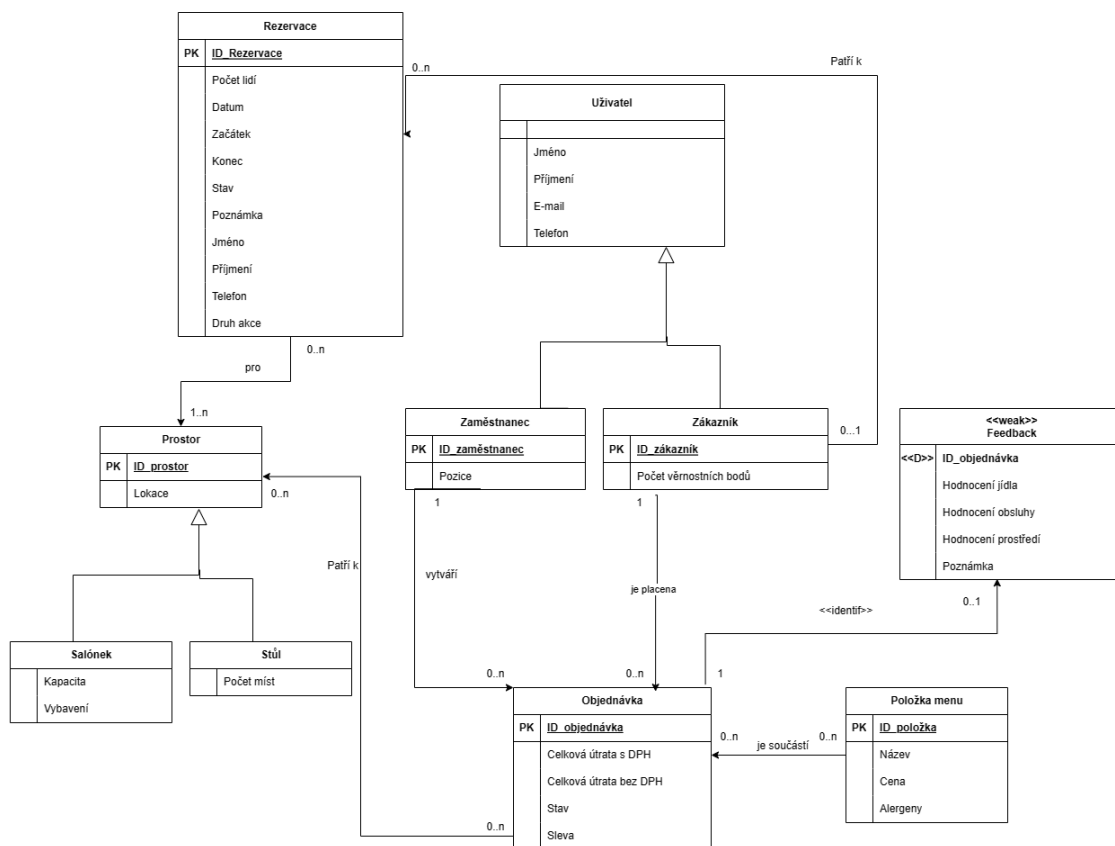
Obrázek 1: Datový model systému pro restauraci
