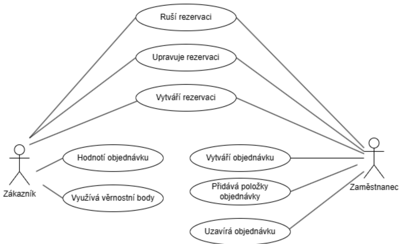
Obrázek 2: Model případu užití systému pro restauraci
